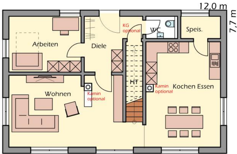
Erdgeschoss Variante 1
